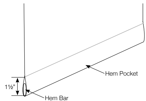
A: OPEN HEM POCKET
