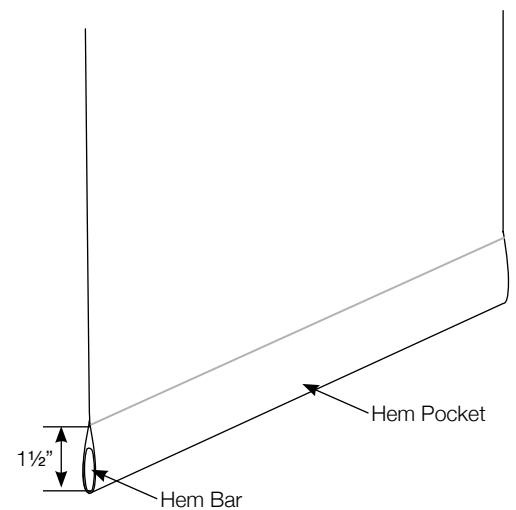
A: OPEN HEM POCKET
